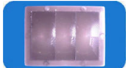
型号：7803- 7 焦距：30 角度：110° 距离：18m 尺寸：25× 32. 5
