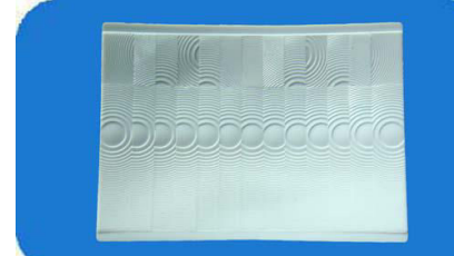
型号: 8720 焦距: 24 角度: 120° 距离: 12m 尺寸: 49×68厚度0.6
