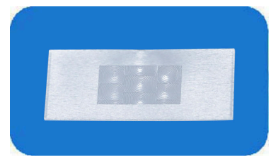
型号: 8501-2D 焦距: 21 角度: 90° 距离: 7m 尺寸: 17.3×42.8
