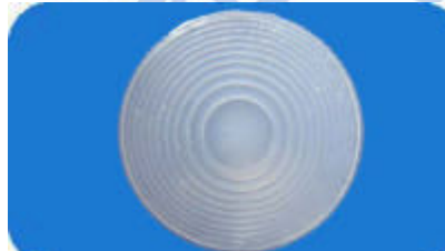
型号：8193 焦距：30 角度：30° 距离比：12: 1 尺寸：Φ 19 厚度: 0. 5
