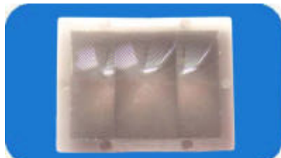
型号：7803- 4 焦距：22. 4 角度：110° 距离：18m 尺寸：25×32. 5
