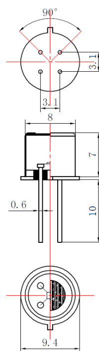
图1 结构及外形尺寸
