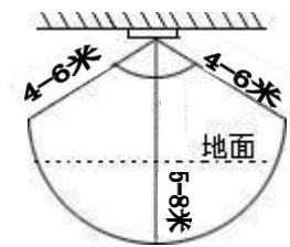
(吸顶安装图示)
